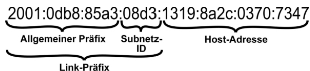
Abb. 1: IPv6-Adresse (Beispiel)
