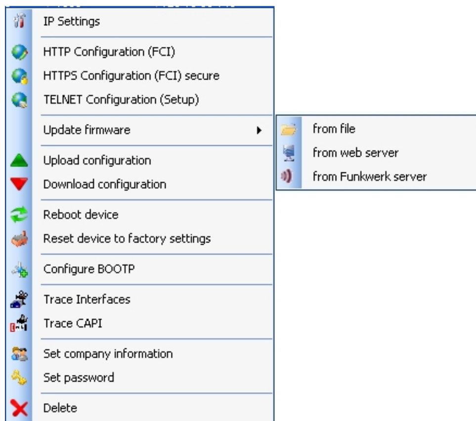
Fig. 7: Shortcut menu
