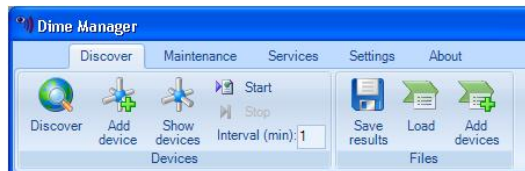
Fig. 3: Menu bar
