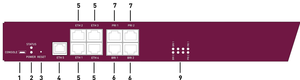
Abb. 9: bintec R4402 Vorderseite
