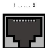
Abb. 17: ISDN-BRI-Schnittstelle (RJ45-Buchse)
