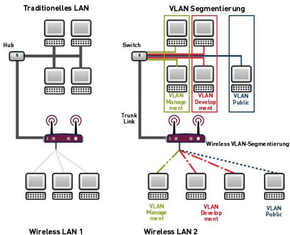
Abb. 59: VLAN-Segmentierung
