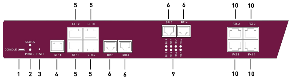
Abb. 10: bintec RT4202 Vorderseite
