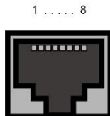
Abb. 16: ISDN-PRI-Schnittstelle (RJ45-Buchse)
