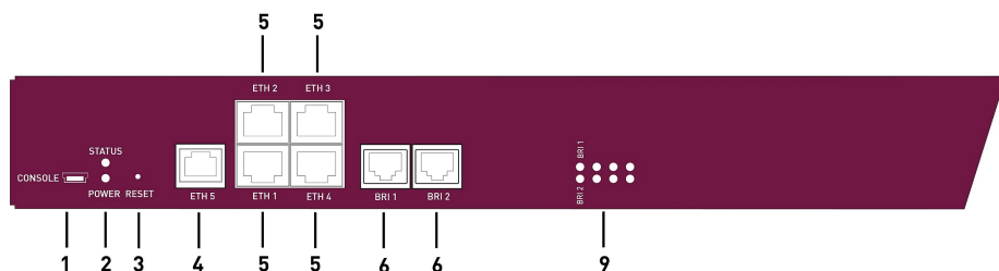
Abb. 6: bintec RT1202 Vorderseite
