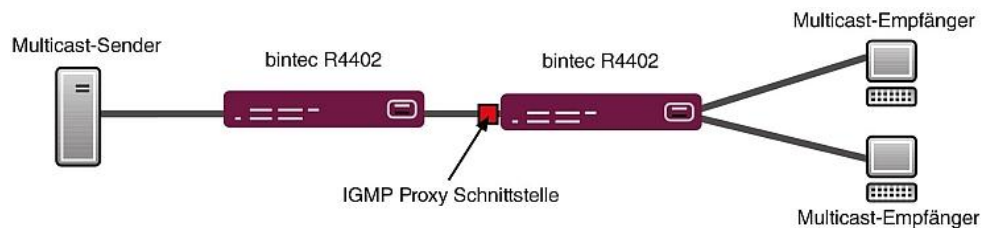
Abb. 109: IGMP Proxy
