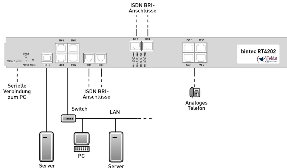
Abb. 2: Anschlussmöglichkeiten am Beispiel bintec RT4202
