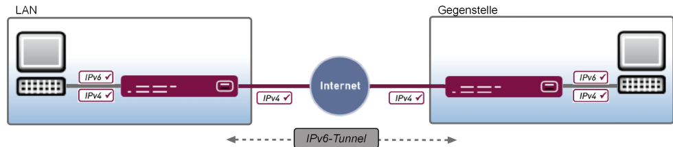
Abb. 123: IPv6-Tunneling-Szenario
