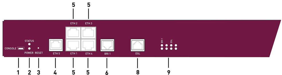
Abb. 7: bintec R3002 Vorderseite
