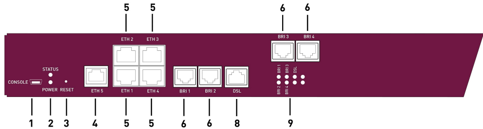
Abb. 8: bintec RT3002 Vorderseite
