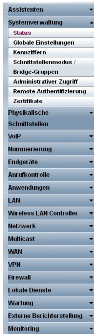
Abb. 24: Menüs
