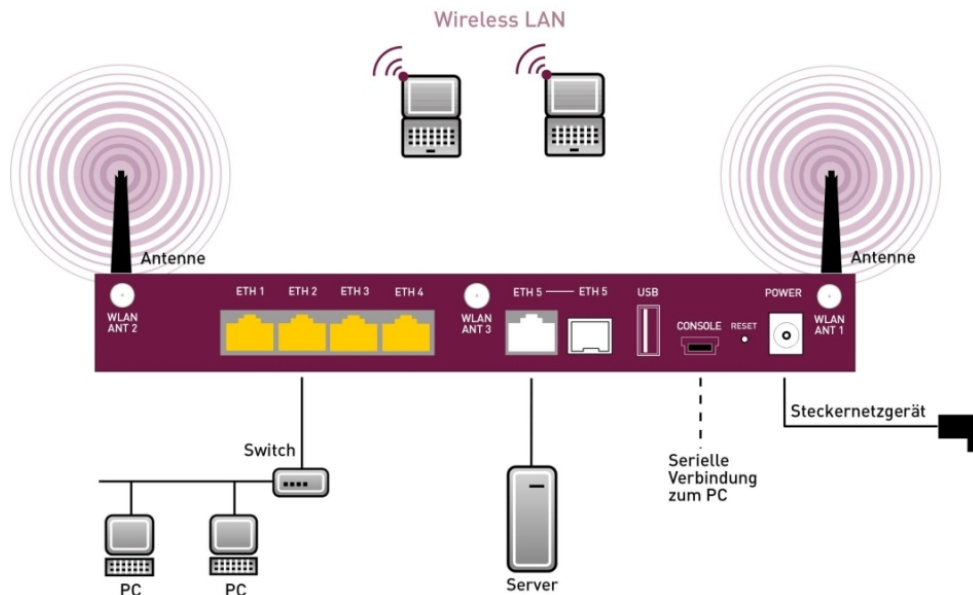
Abb. 2: Anschlussmöglichkeiten am Beispiel bintec RS120wu
