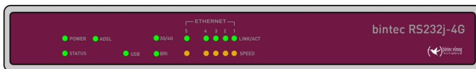
Abb. 16: Anordnung der LEDs
