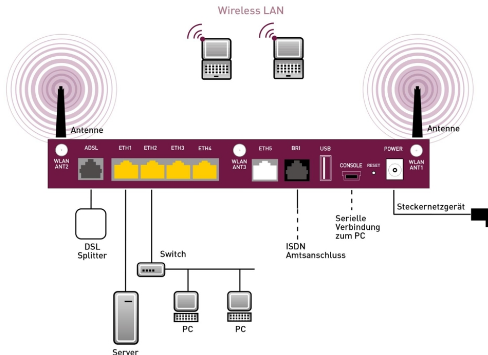
Abb. 12: Anschlussmöglichkeiten am Beispiel bintec RS232jw
