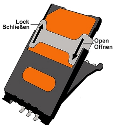
Abb. 22: SIM-Karte
