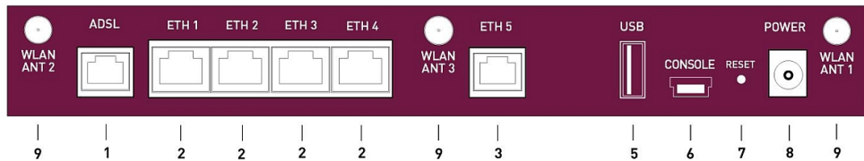
Abb. 8: bintec RS230aw Rückseite
