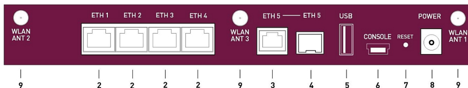
Abb. 3: bintec RS120wu Rückseite
