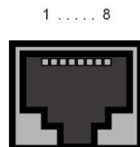
Abb. 20: ISDN-S0 -BRI-Schnittstelle (RJ45-Buchse)
