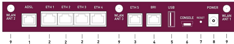
Abb. 13: bintec RS232jw Rückseite
