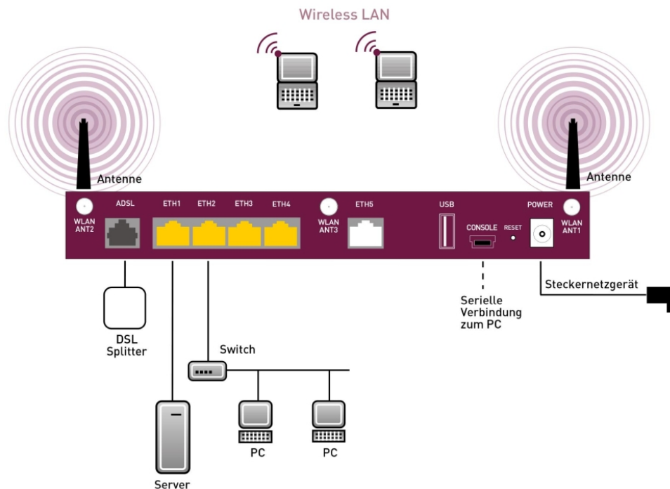
Abb. 7: Anschlussmöglichkeiten am Beispiel bintec RS230aw
