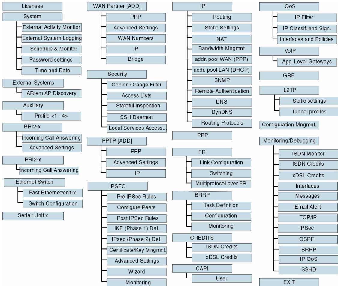
Abbildung 4-3: Setup-Tool-Menüstruktur
