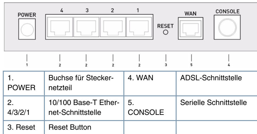
Abbildung 1-2: X2301 Rückseite
