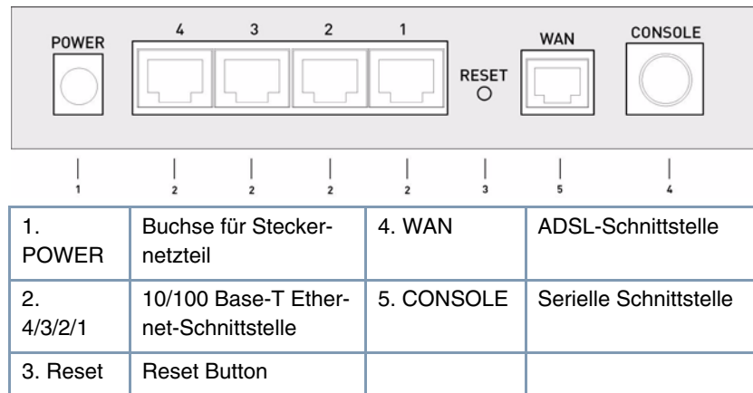
Abbildung 2-2: X2302 Rückseite
