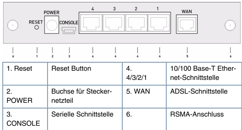
Abbildung 2-2: X2302w Rückseite
