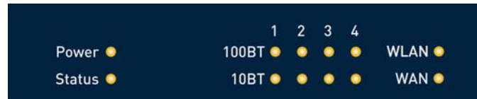
Abbildung 2-1: LEDs von X2302w
