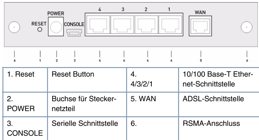
Abbildung 1-2: X2301w Rückseite
