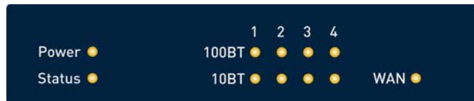
Abbildung 2-1: LEDs von X2302
