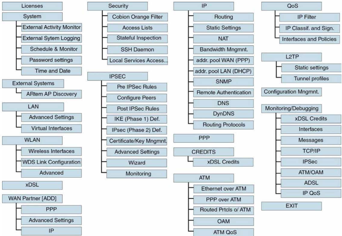
Abbildung 4-2: Setup-Tool-Menüstruktur
