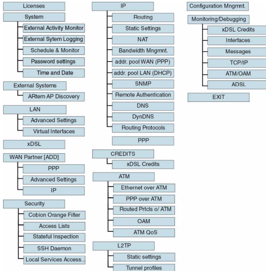
Abbildung 4-2: Setup-Tool-Menüstruktur
