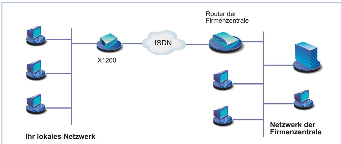
Bild 3-4: X1200 in Ihrer Niederlassung
