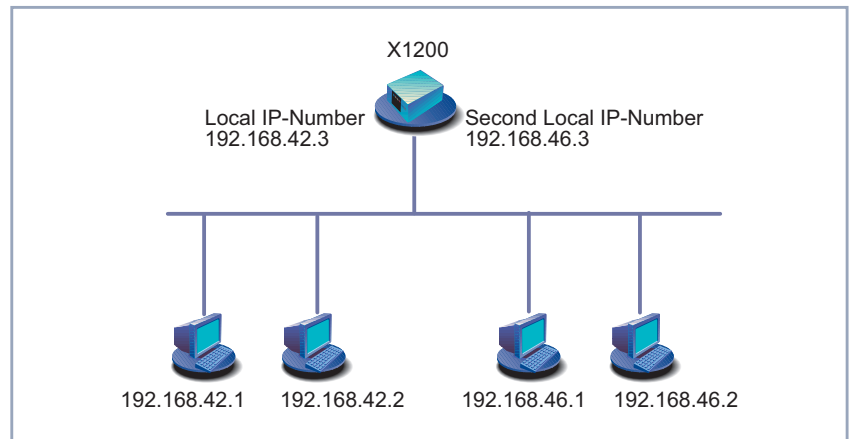
Bild 6-2: X1200 mit zwei verschiedenen lokalen IP-Adressen
