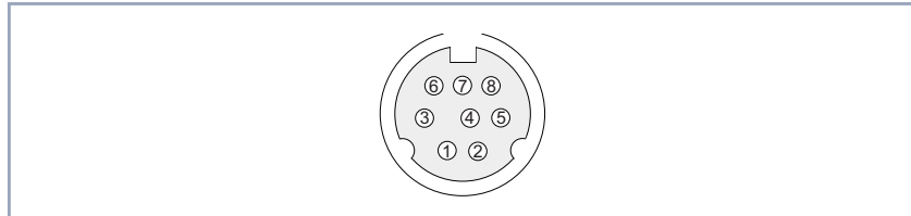
Bild 11-3: 8-polige MiniDin-Buchse
