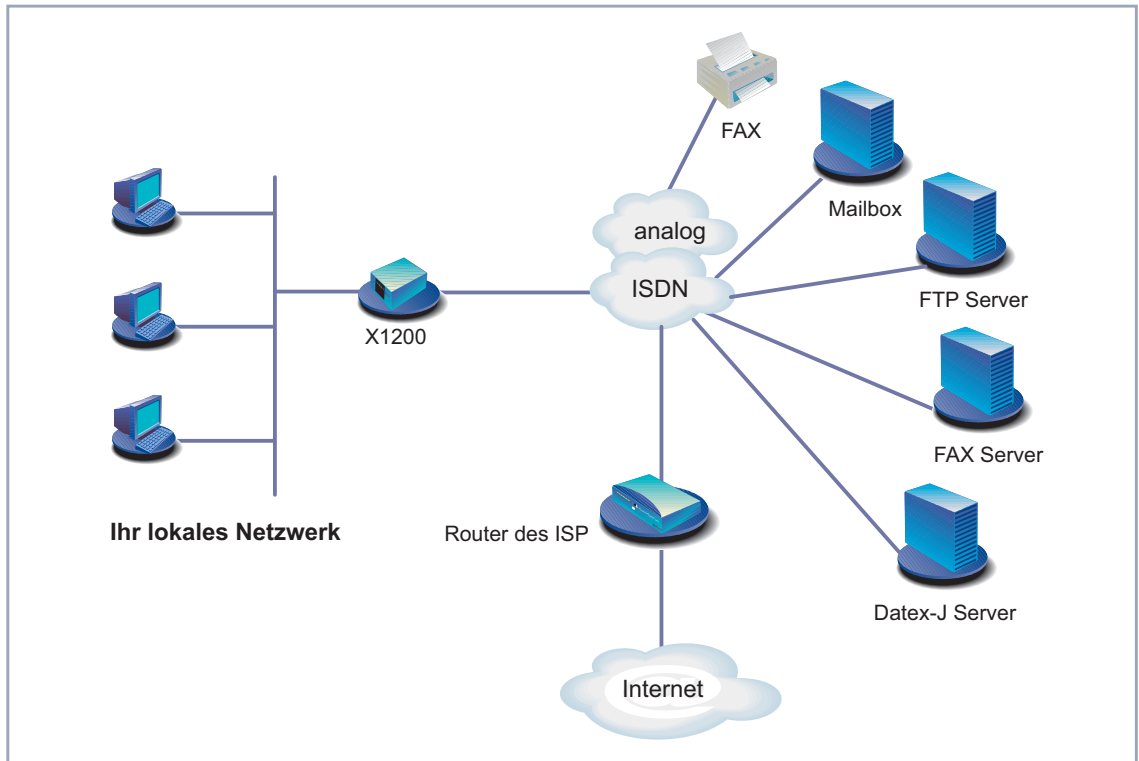
Bild 3-3: X1200 mit Kommunikationsanwendungen
