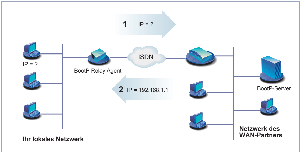
Bild 7-4: X1200 als BOOTP-Relay-Agent
