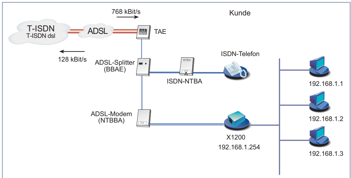
Bild 3-2: T-ISDN-dsl-Anschluß
