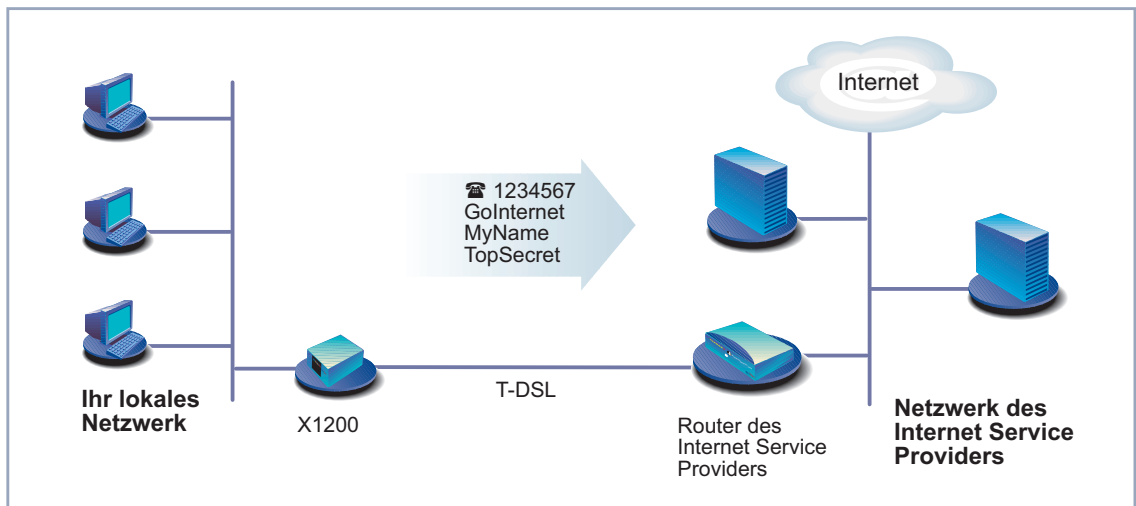
Bild 3-10: X1200 und Ihr Internet Service Provider
