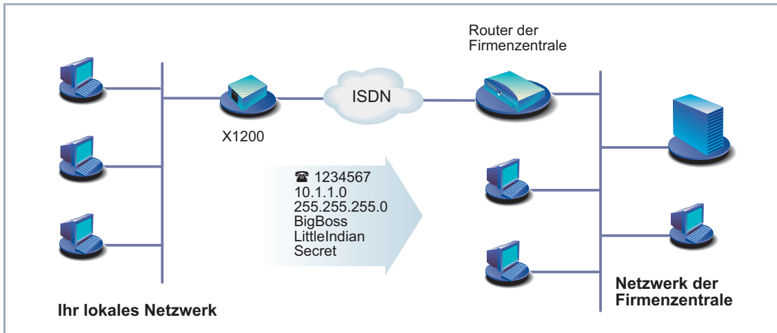
Bild 3-11: X1200 und Ihre Firmenzentrale
