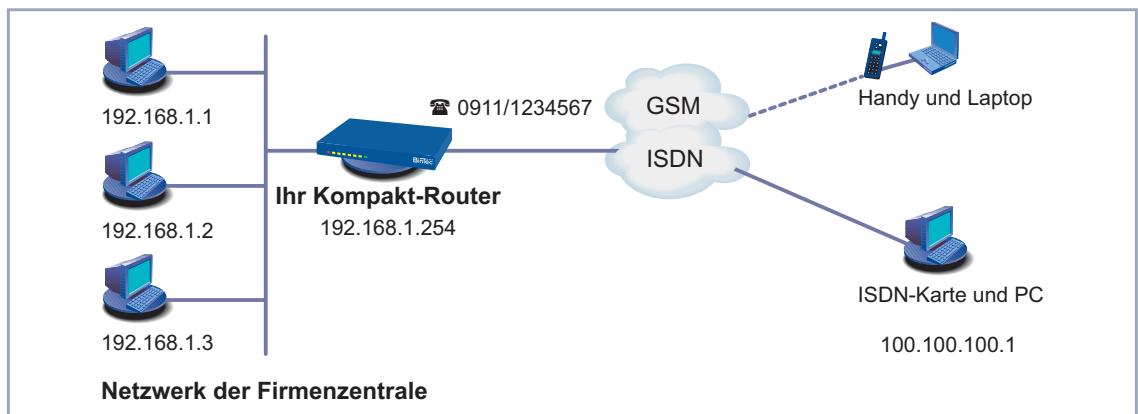
Bild 6-7: Szenario für Dial-in
