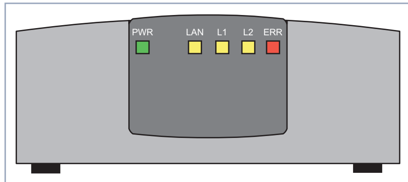
Bild 8-1: X1000 : Vorderseite
