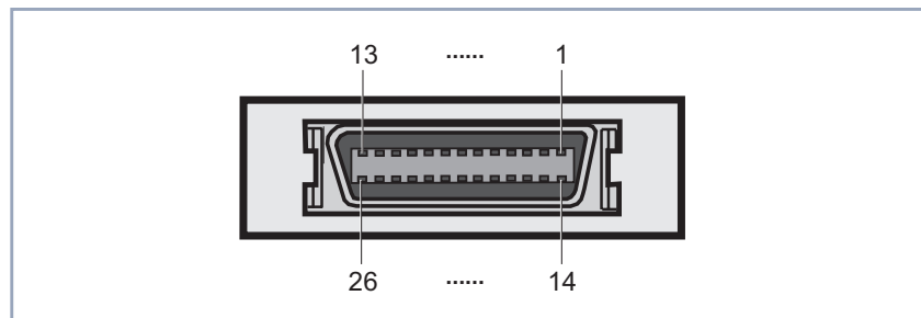
Bild 8-22: 26-polige Mini-Delta-Ribbon-Buchse
