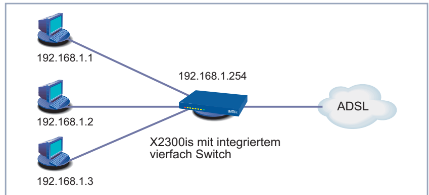
Bild 4-3: Rechner direkt an X2300is
