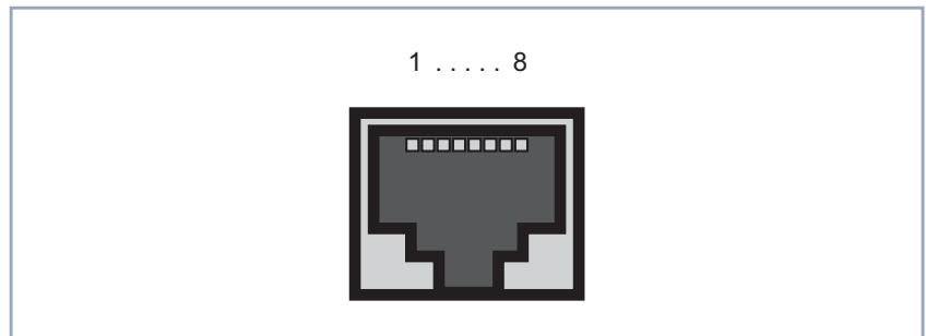
Bild 8-18: ISDN-S 0 -BRI-Schnittstelle (RJ45-Buchse)
