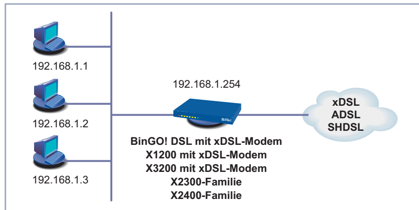
Bild 4-2: DSL-Anschluß
