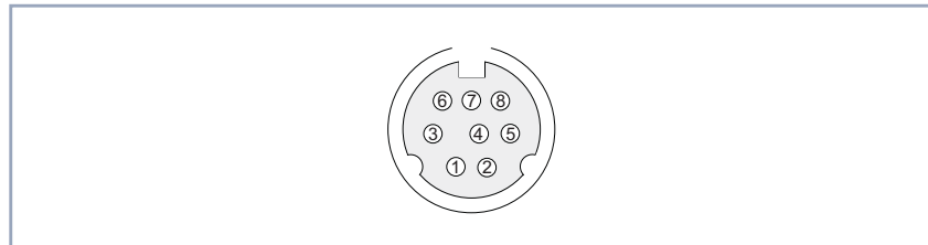
Bild 8-17: 8-polige MiniDin-Buchse
