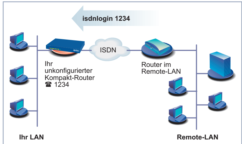
Bild 5-2: Zugang über ISDN-Login für Fernwartung
