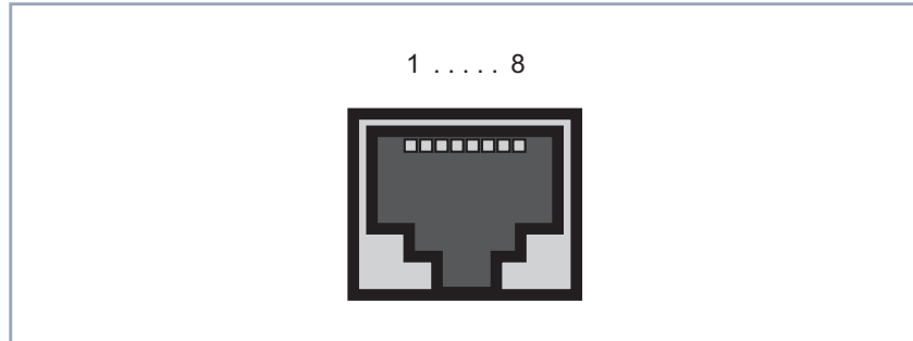
Bild 8-24: ADSL-Schnittstelle von X2300 (RJ45-Buchse)
