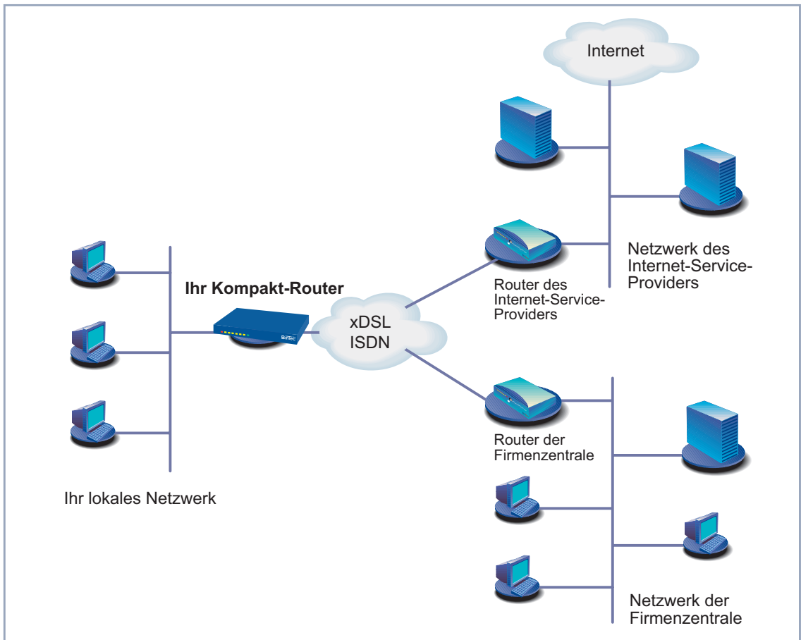
Bild 1-1: Grundszenario für Kompakt-Router von BinTec
