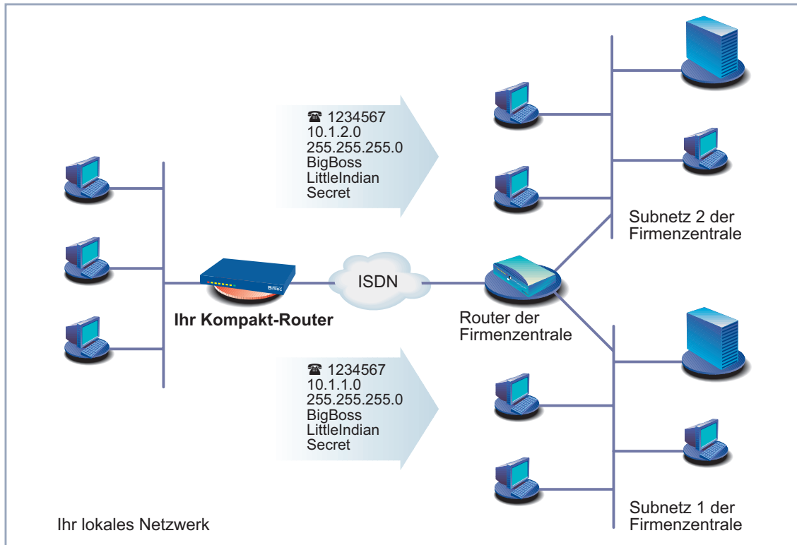
Bild 6-5: Netzwerk mit Subnetzen
