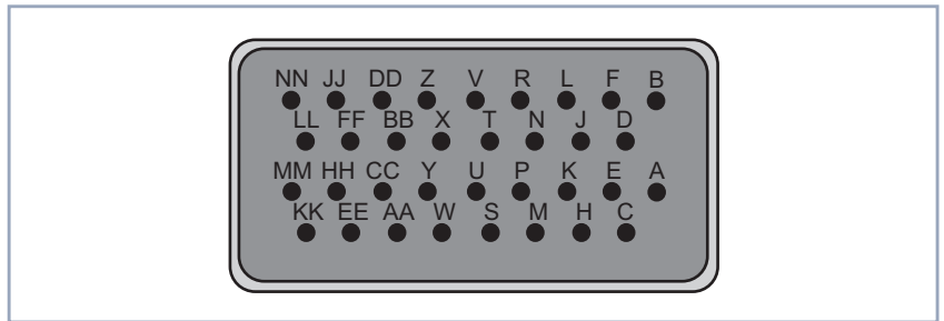
Bild 8-21: M34-Stecker
