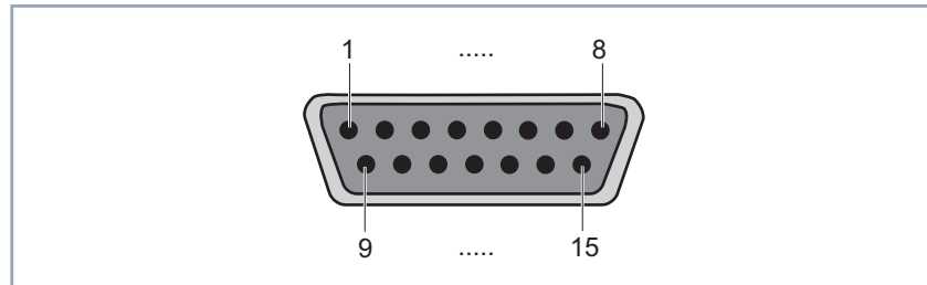
Bild 8-20: DB-15-Stecker (DTE)
