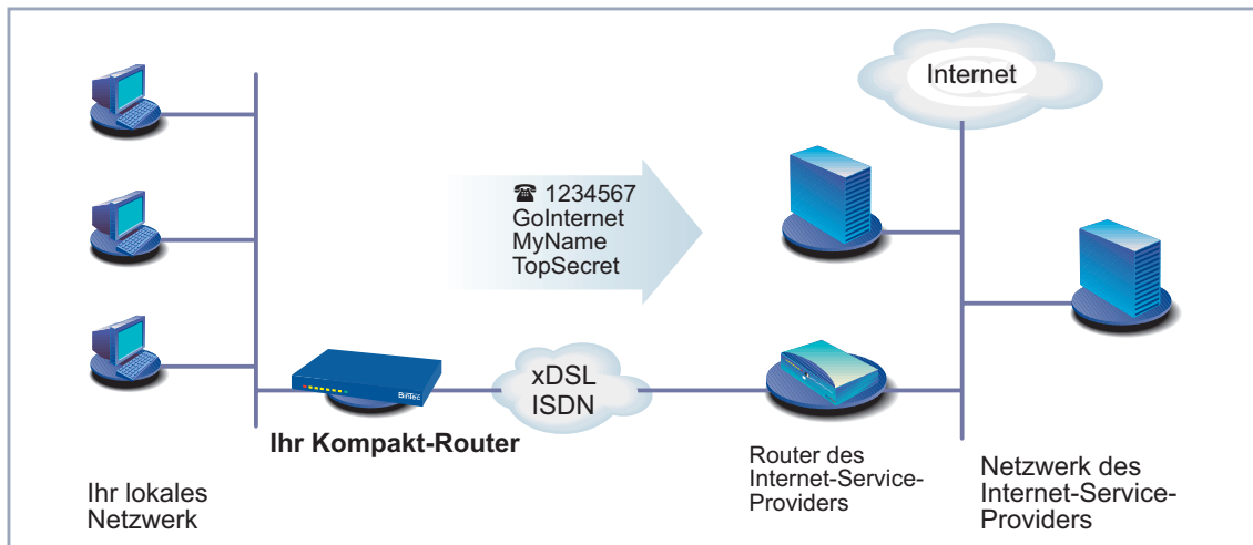
Bild 4-1: Die ISDN-Schnittstelle Ihres BinTec-Kompakt-Routers und Ihr Internet-Service-Provider
