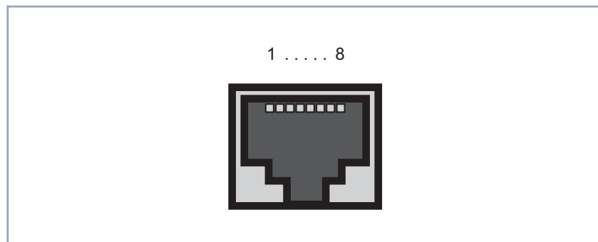
Bild 8-26: SHDSL-Schnittstelle von X2404 (RJ45-Buchse)
