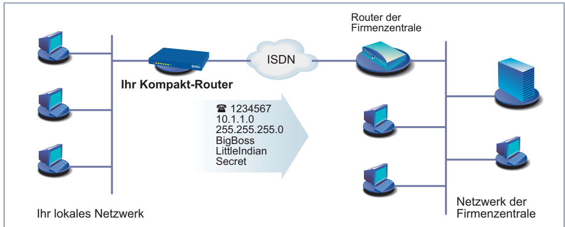
Bild 4-5: Ihr BinTec-Router in der Niederlassung
