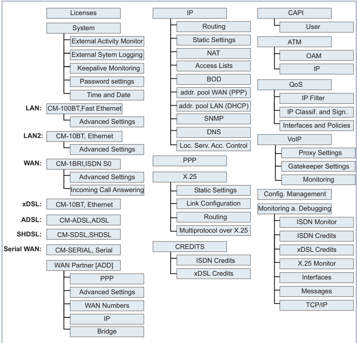
Bild 5-4: Setup-Tool-Menüstruktur
