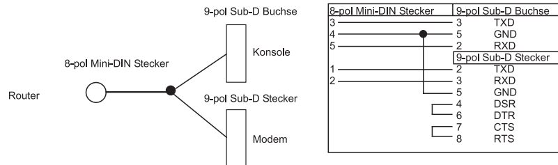
Abbildung 1-2: Spezifikation Zweifach-Modemkabel
