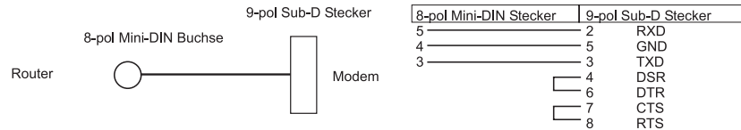
Abbildung 1-1: Spezifikation Einfach-Modemkabel
