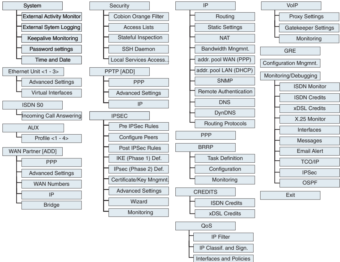
Abbildung 4-2: Setup-Tool-Menüstruktur
